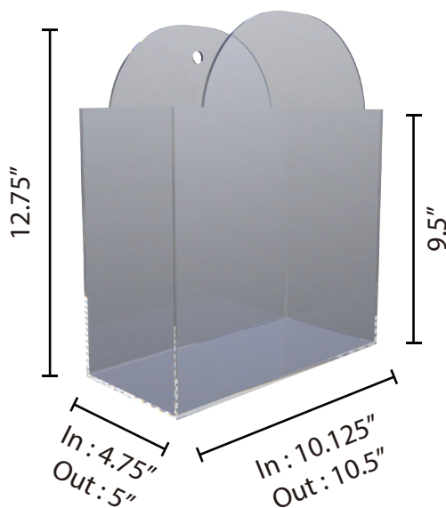
Catalog Holder
